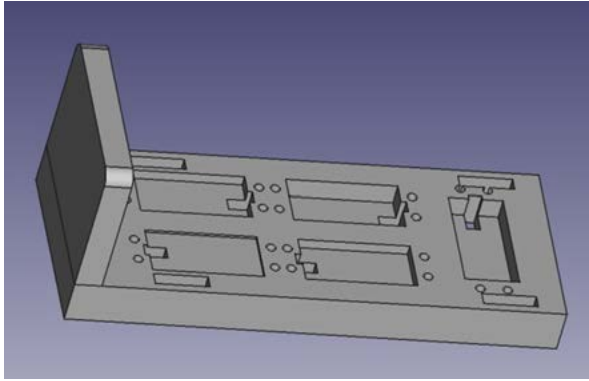
Fig. 4. Brazaete de la órtesis con espacios para los servomotores con distintas alturas para evitar rozamiento del filamento.
