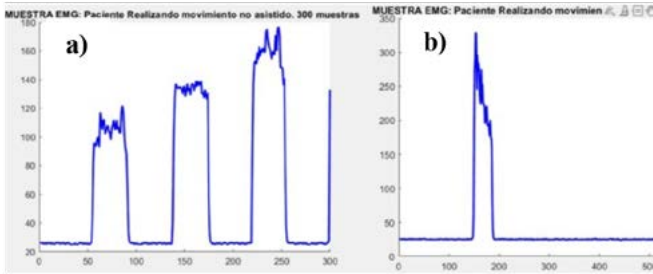
Fig. 8. Actividad muscular flexora; a) actividad muscular del flexor de las falanges proveniente del movimiento voluntario del paciente; b) actividad muscular del flexor cuando el paciente hace uso del dispositivo.
