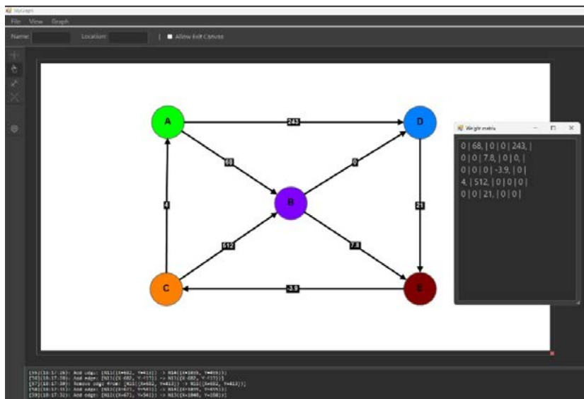
Fig. 18. Ejemplo de una matriz de pesos usando el grafo ponderado dirigido de la figura 9.
