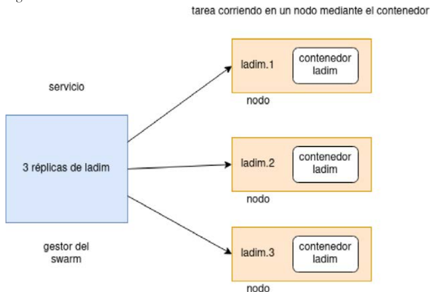
Fig. 7. Funcionamiento de docker swarm.
