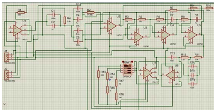
Fig. 3. Diagrama esquemático del circuito EMG.
