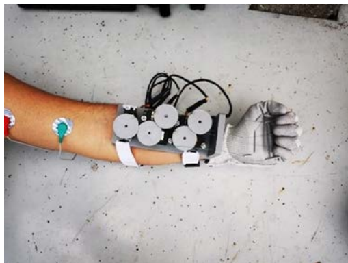
Fig. 10. Estado de contracción con EMG de la órtesis.
