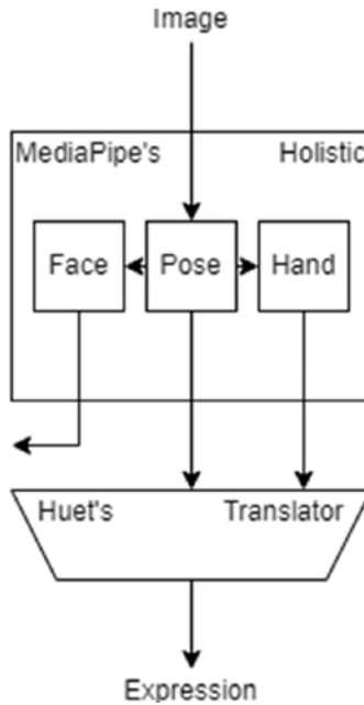
Fig. 10. Funcionamiento de Holistic y Translator
