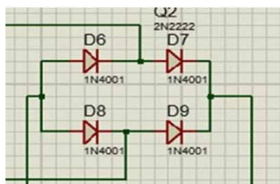
Fig. 8. Puente rectificador.
