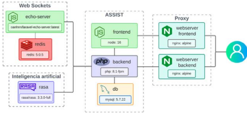
Fig. 7. Diagrama ilustrativo de la arquitectura y comunicación de los servicios del sistema.
