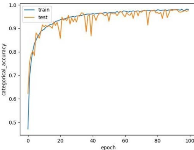
Fig. 11. Precisión del traductor.
