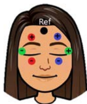
Fig. 2. Distribución de los siete electrodos para registrar los movimientos oculares de los tres canales involucrados: derecho (electrodos rojos), izquierdo (electrodos azules) y laterales (electrodos verdes), así como la referencia (electrodo negro).
