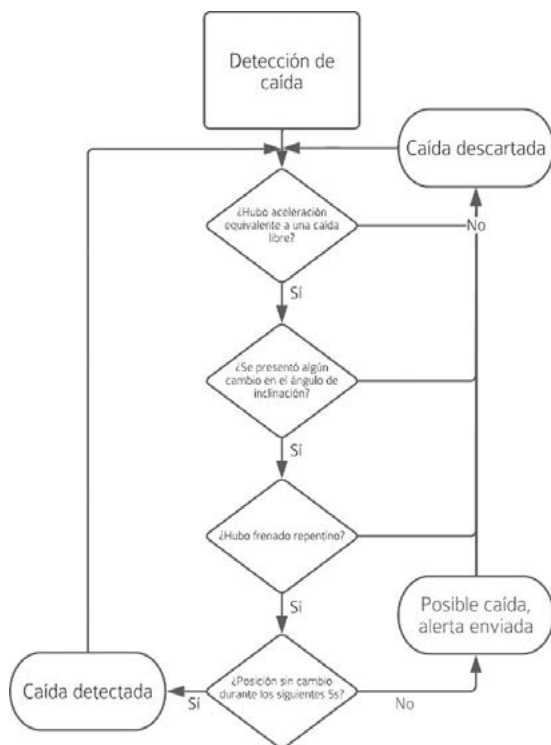
Fig. 1. Diagrama de secuencia detección de caídas.
