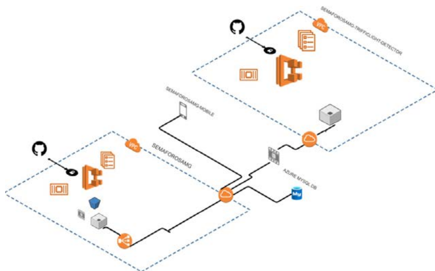
Fig. 2. Diagrama de componentes que representa la arquitectura implementada del sistema. Se mencionan los recursos utilizados en la elaboración del mismo.
